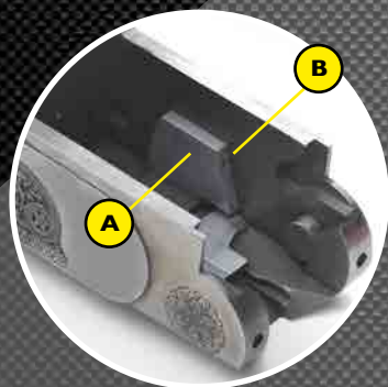
Particolare del tassello intercambiabile sul rampone A. Tassello estraibile B. Spina di fermo
