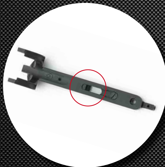
Particolare del dispositivo di autotensionamento della croce. Details of self tension on the iron forend
